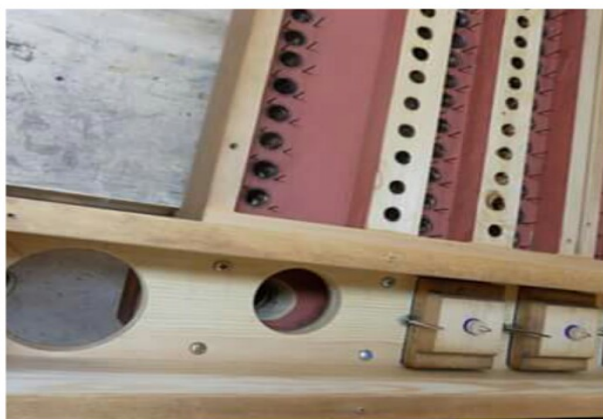
vzdušnica I. manuálu pred opravou
